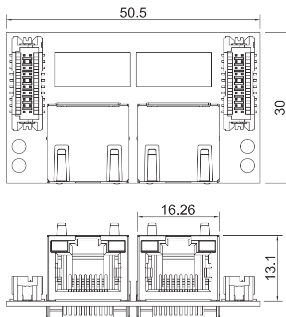
LAN I/O Card
